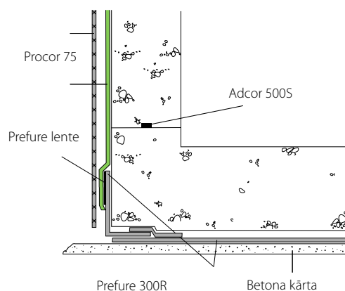
Ārēja bituma izolācijas veidošana uz betona apakšbūves
